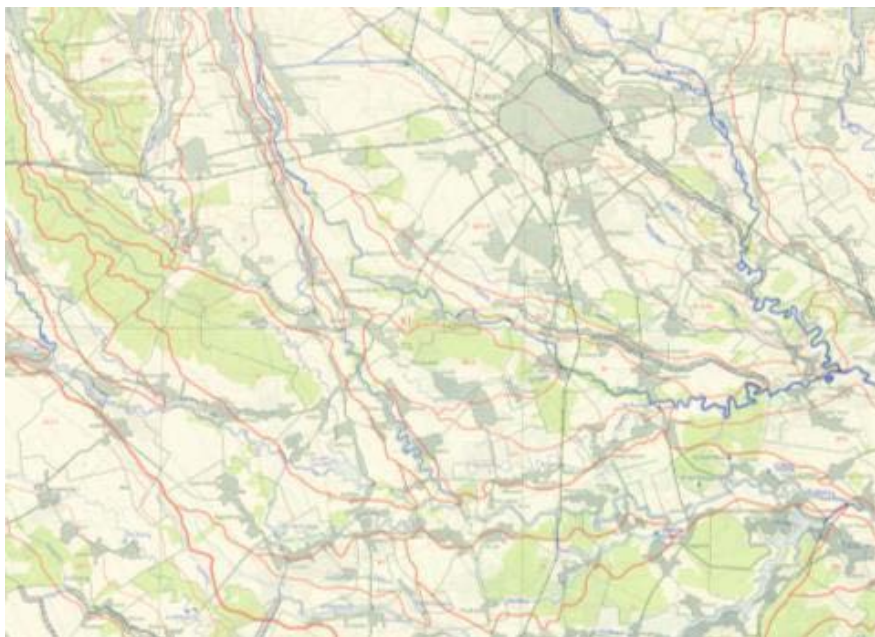
Figura 44 – Harta hidrologică a zonei [Raport de amplasament Veolia, 2017]
