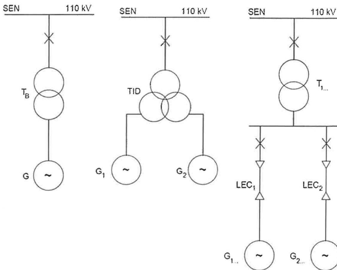
Fig. 3.14 – Soluții de racordare a grupurilor generatoare la noduri electrice
