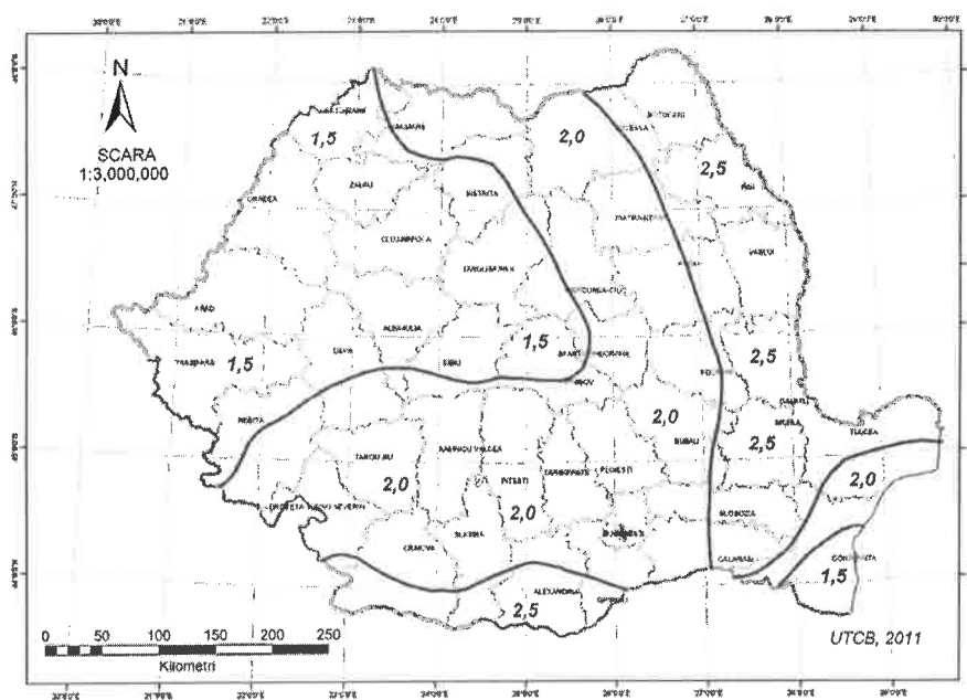
Figura 3.1 Zonarea valorilor caracteristice ale încărcării din zăpadă pe sol s_k , \text{kN/m}^2 , pentru altitudini A \leq 1000 \text{ m} Notă: Pentru altitudini A > 1000 \text{ m} valorile s_k se determină cu relațiile (3.1) și (3.2)
